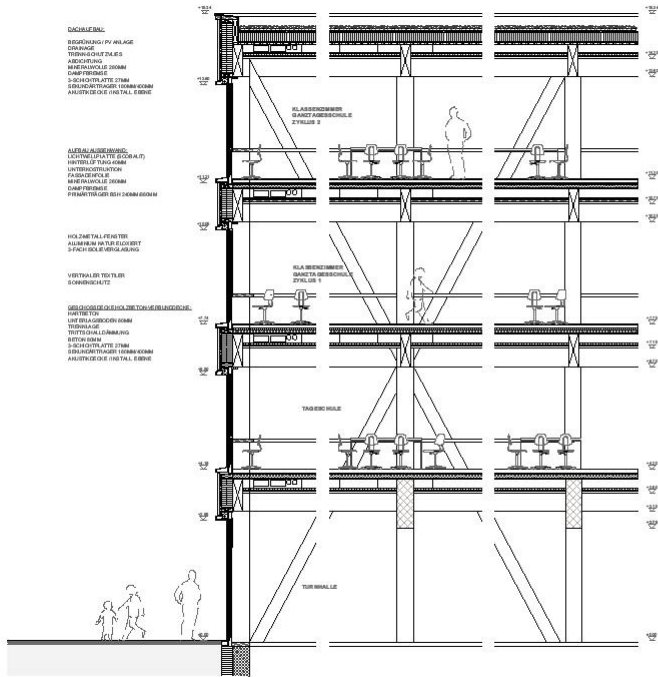
DETAILSchnitt Gebäudehülle 1:50
