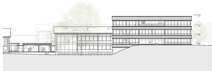
ANSICHT SÜDOST 1:200
