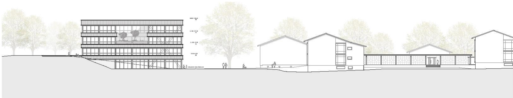
ANSICHT NORDOST 1:200
