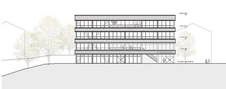
ANSICHT NORDWEST 1:200
